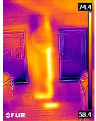
دیوار میں گرم ڈرین پائپ
